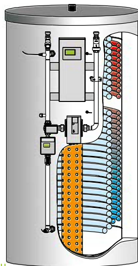
HPDL-H mit Ultraschall-Wärmemengenzähler
