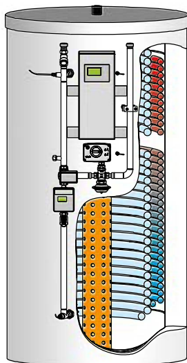
HPZL-H mit Ultraschall-Wärmemengenzähler
