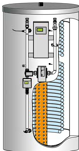
SPDL-H mit Ultraschall-Wärmemengenzähler
