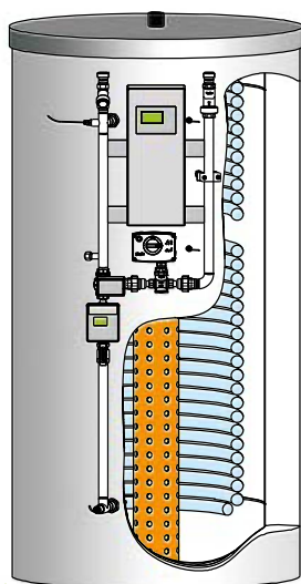
SPZL-H mit Ultraschall-Wärmemengenzähler
