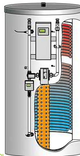
HPDL mit Ultraschall-Wärmemengenzähler
