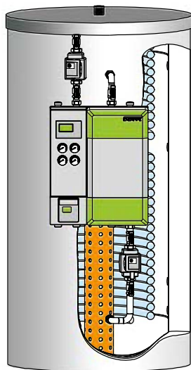
ÜPDL-H mit Ultraschall-Wärmemengenzähler
