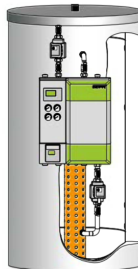
ÜPDL mit Ultraschall-Wärmemengenzähler
