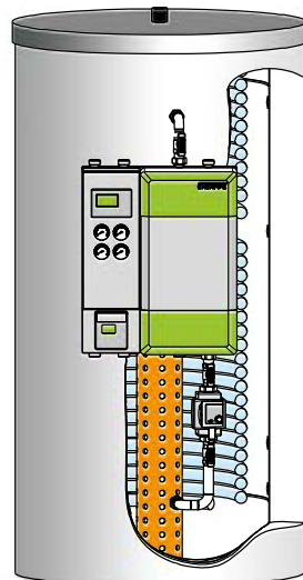
ÜPZL-H mit Ultraschall-Wärmemengenzähler
