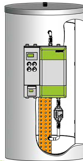
ÜPZL mit Ultraschall-Wärmemengenzähler
